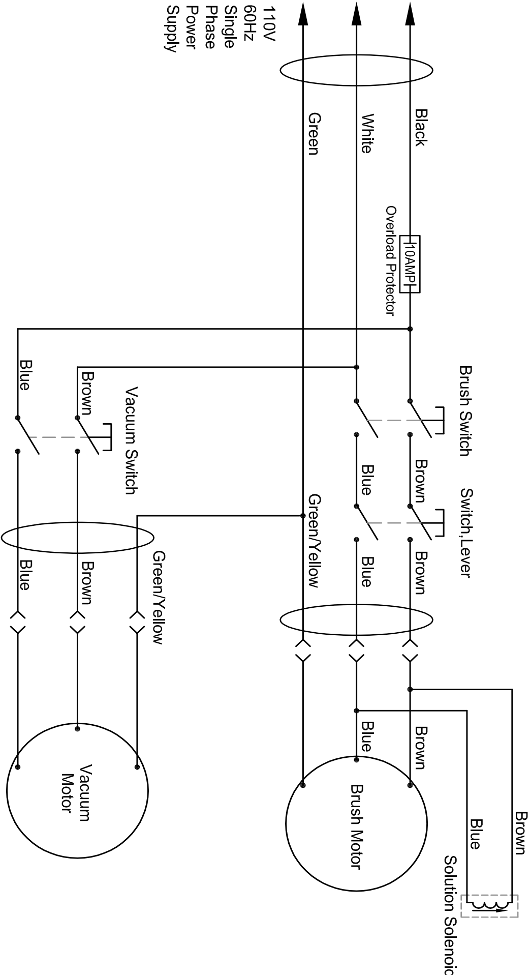
WIRING DIAGRAM(i18C)
